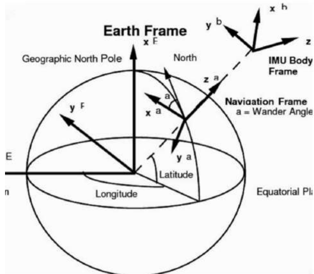
Earth's latitude and longitude coordinate system.
